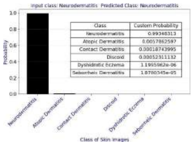
Fig.8(d).ProbabilitiesofClasses
