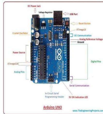
Fig.2. Arduino UNO
